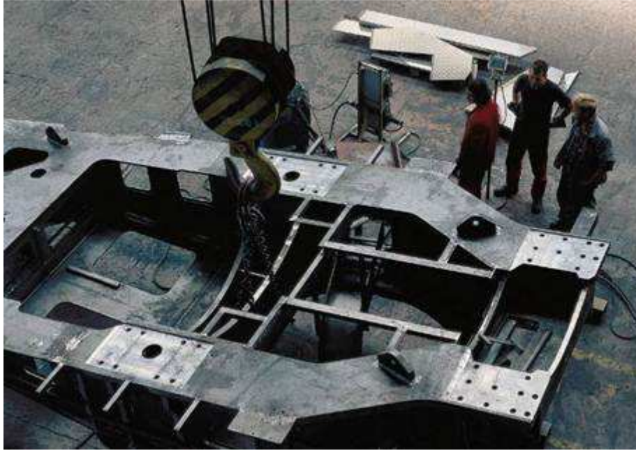
Nosný rám stroje větrné elektrárny
