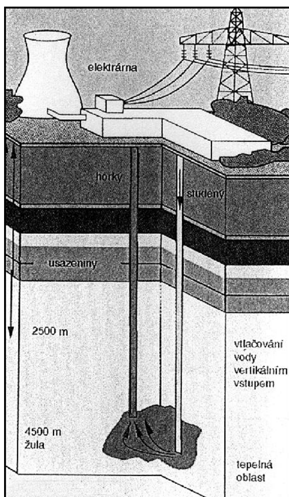
Geotermální elektrárna
