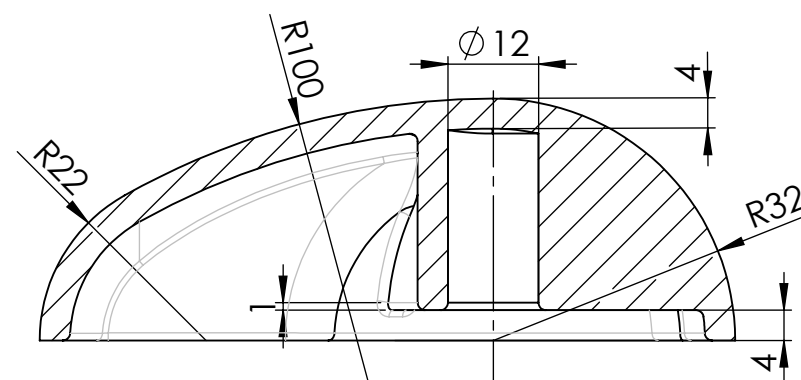
ŘEZ A-A
