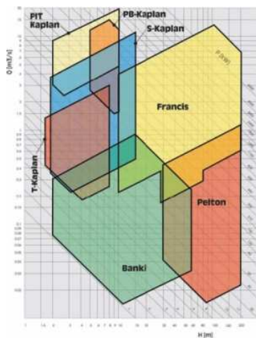
Základní charakteristika turbín podle průtoku a spádu. © EkoWATT
